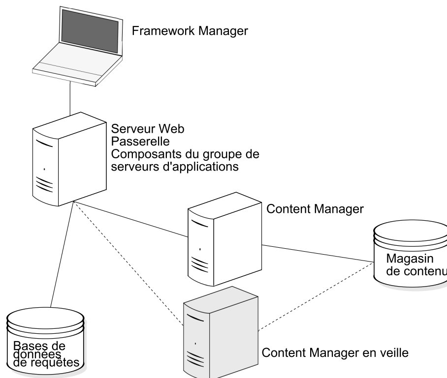
Figure 3. Installation avec un ordinateur Content Manager actif et un ordinateur Content Manager de secours
