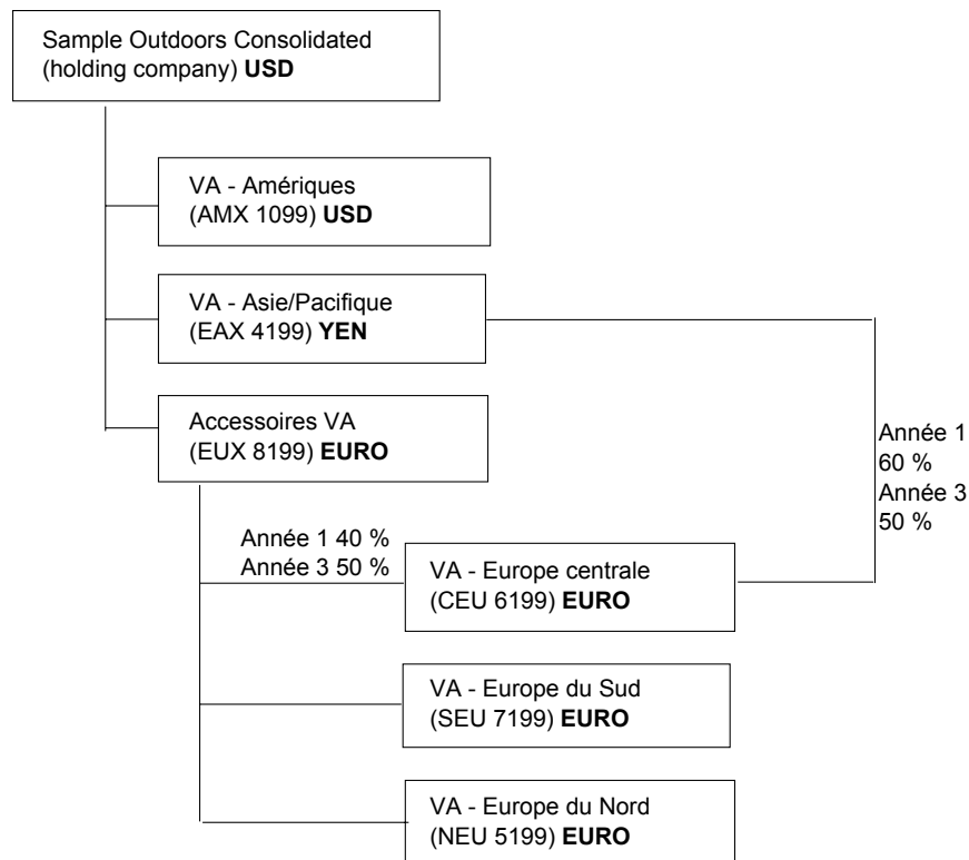
Figure 13. Structure d'organisation consolidée
