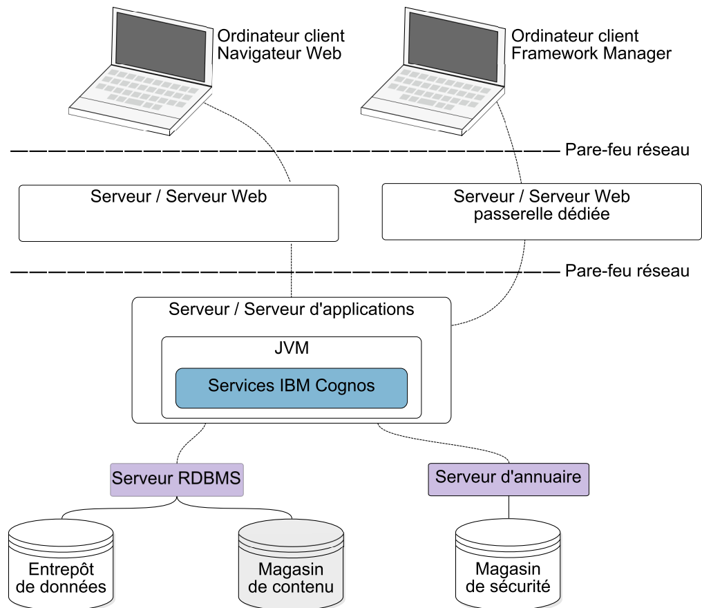
Figure 7. Ordinateur client à l'extérieur du pare-feu
