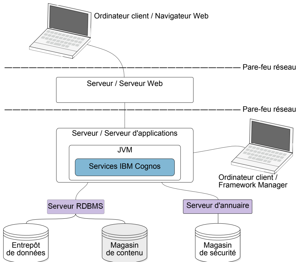
Figure 6. Ordinateur client à l'extérieur du pare-feu
